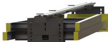
Interner Leiterhalter
